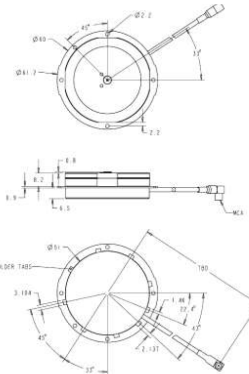
TW3870E Dimensions (mm)
